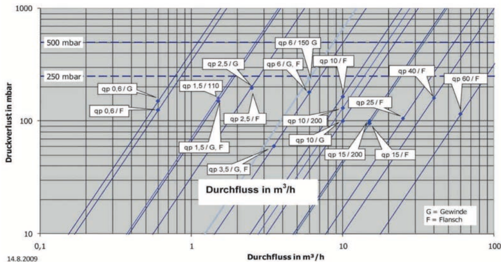
Druckverlust 2WR7
