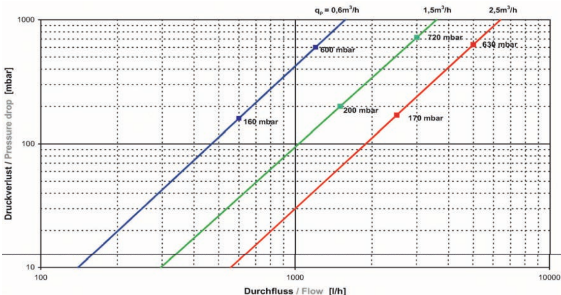
Druckverlustdarstellung des Einstrahl-Kompaktwärmemengenzählers "Calidus-tec"
