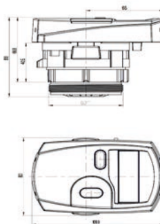
"Plus"-Messkapsel mit splitbarem Rechenwerk
